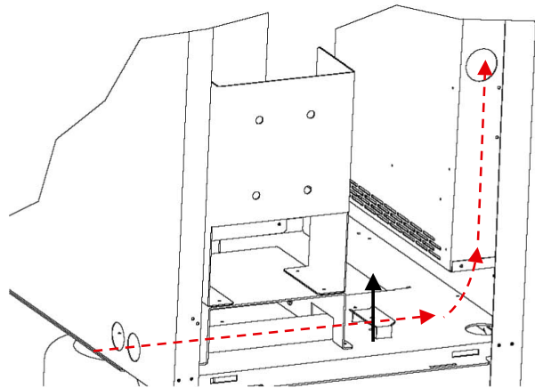
Das Netzkabel ist durch die Führungsrohre seitlich in den Schaltkasten zu führen und mit der Zugentlastung zu sichern.
